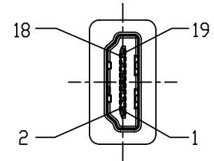
HDMI 19-F
