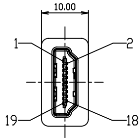
HDMI 19-F
